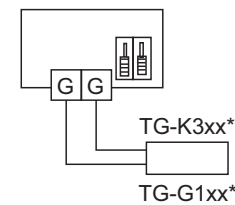
Положение переключателя и схема подключений при использовании внешнего датчика и задатчика уставки
